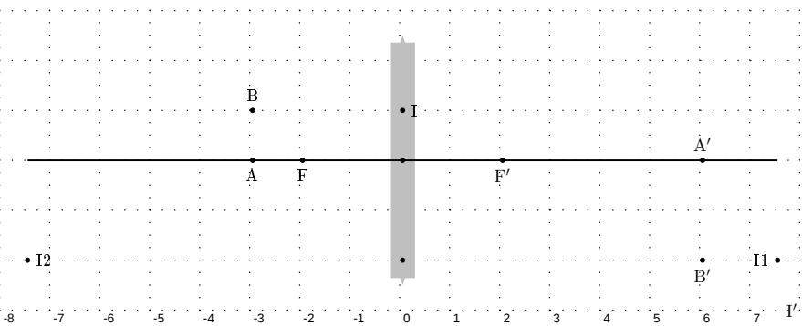
Abbildung 1: Die Lage der von pst-optic vordefinierten Knotenpunkte für Sammel- und Zerstreuungslinse mit Bezeichnungen
