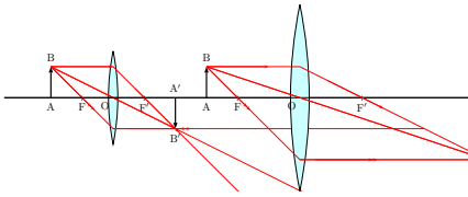
(a) Definition zweier unabhängiger Linsen
