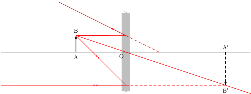
Abbildung 3: \lens[lensType=DVG] (Zerstreuungslinse)
