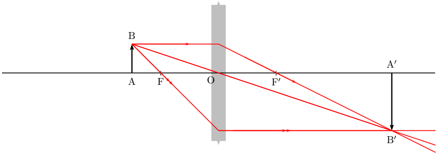
Abbildung 2: \lens[lensType=CVG] (Sammellinse)
