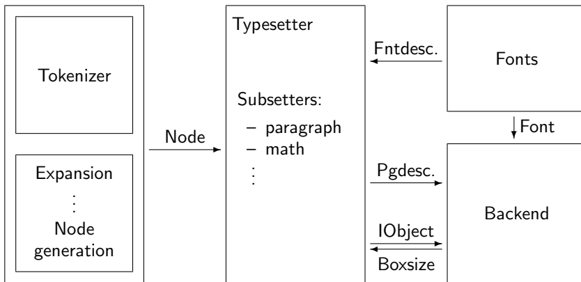
Abbildung 1: Primäres Komponenten-Design von \epsilon\lambda\text{T}_{\text{E}}\text{X}
