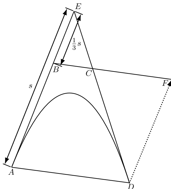
Abbildung 1: Visualisierung von quadratischen Bézier-Kurven (Parabeln)
