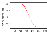
Abb. 4: Die approximierte AP-VS-Kennlinie als Funktion der Herzfrequenz.
