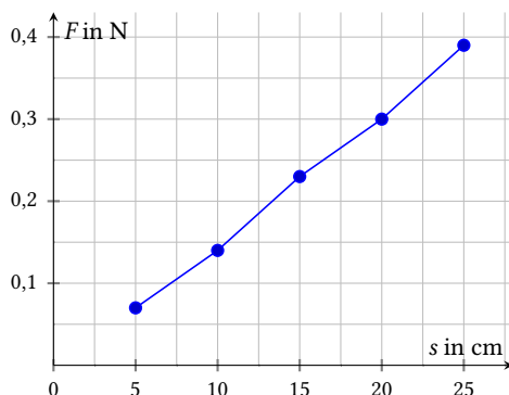
Abb. 8: Koordinatensystem mit Messpunkten
