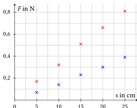
Abb. 10: Koordinatensystem mit zwei Messreihen
