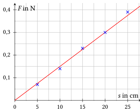
Abb. 13: Ursprungsgerade mit manuell festgelegter Gleichung
