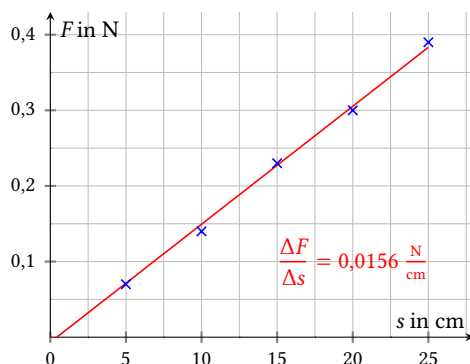
Abb. 12: Regressionsgerade mit formatierter Ausgabe der Steigung
