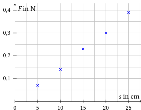
Abb. 9: Koordinatensystem mit unverbundenen Messpunkten
