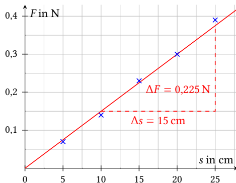
Abb. 14: Ursprungsgerade mit Steigungsdreieck
