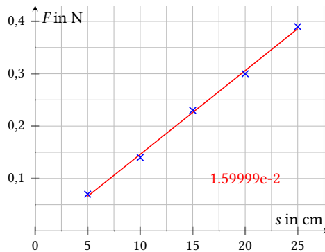
Abb. 11: von pgfplots berechnete Regressionsgerade mit Steigung
