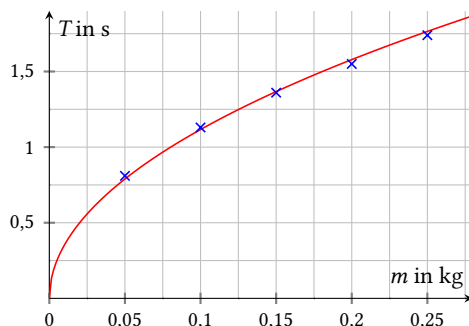
Abb. 15: Messreihe mit Ausgleichskurve
